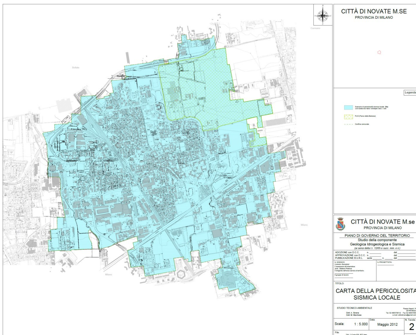
Immagine – Pericolosità Sismica Locale – Classificazione di Novate Milanese
